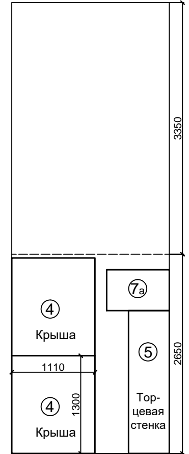
Лист 3 2.1x2.65 м
